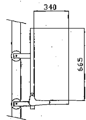
荷台(折畳式)
